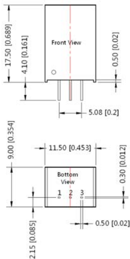
K78XX
